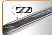
Patentovaný U profil držadla
